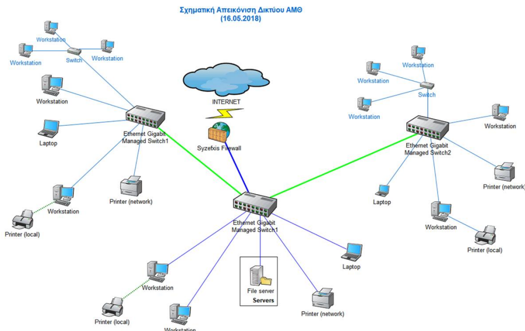
Σχηματική απεικόνιση δικτύου ΑΜΘ
